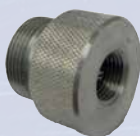
Adapter GA-HT-A1 utv M28x1,5 x 1615
